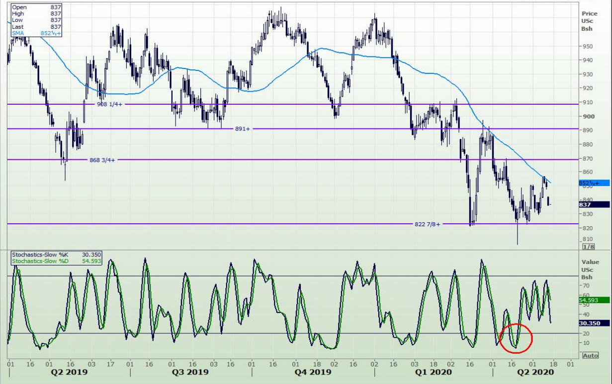
Daily SOYBEANS MAYO
